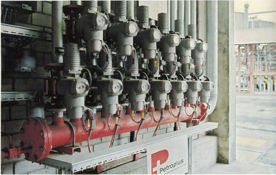
Abb. 5: Absperr-Kugelhähne der Franz Gysi AG mit montiertem Elektroantrieb in einer Brandschutzanlage eines Mineralöl-Lagers. Die Armaturen werden im Brandfall ferngesteuert geöffnet, damit Löschschaum und Wasser ausströmen können.
