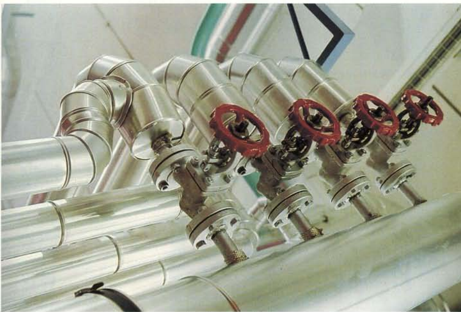
Abb. 6: Absperr-Ventile der Franz Gysi AG an einem Dampf-Kessel in einer Industrie-Anlage. Mit den Ventilen wird die Dampf-Verteilung geregelt. Die Armaturen müssen gleichzeitig hohem Druck und hohen Temperaturen standhalten.
